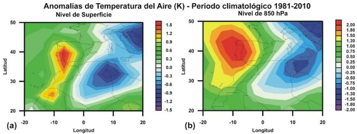
Figura 32. Mapas sinópticos promedio compuestos a partir de datos de anomalías de temperatura a nivel de superficie (a) y en el nivel de 850 hPa (b) durante los días de evento de combustión de biomasa en 2004-2009.
