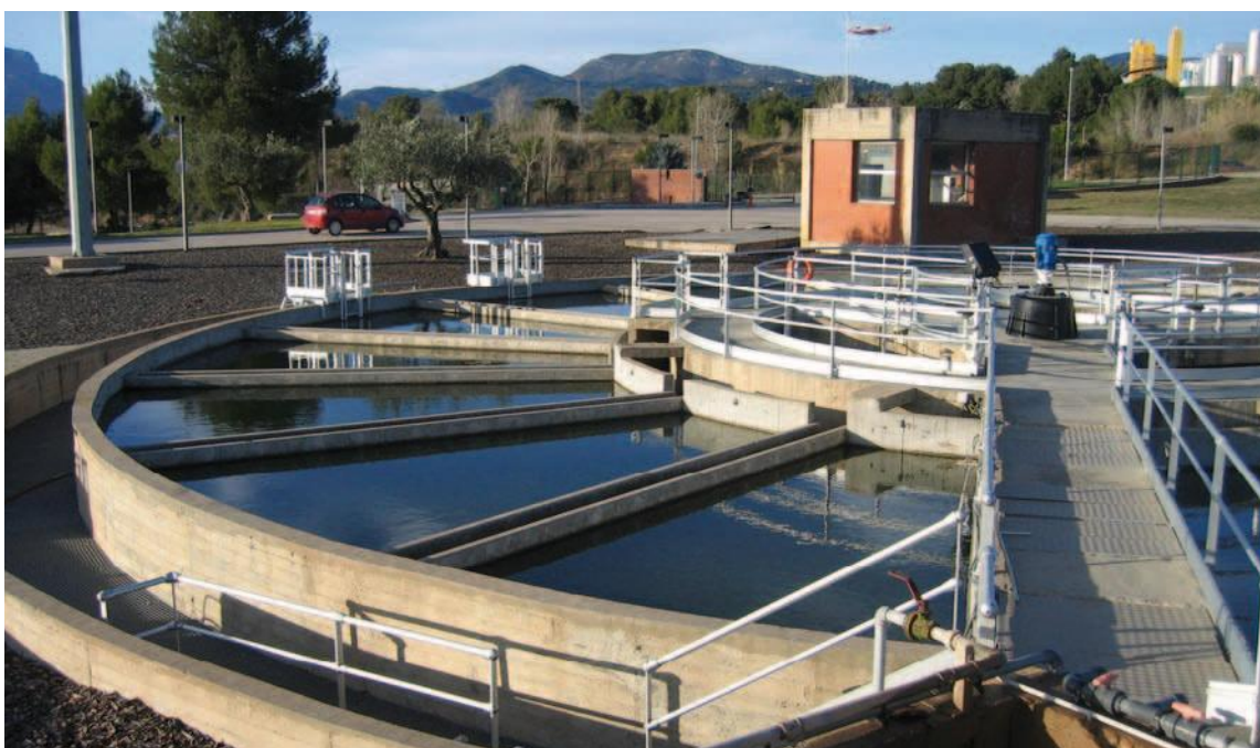
Figura 10. Planta de potabilización de Abrera. Aguas Ter Llobregat. Barcelona
